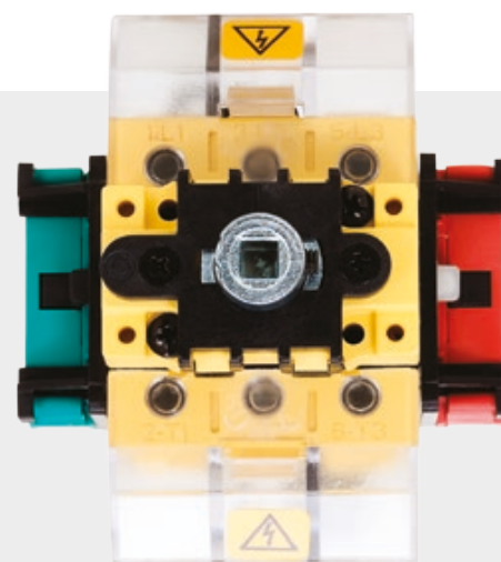
Exemplo de chave com 2 contatos auxiliares e 2 cobre bornes.
